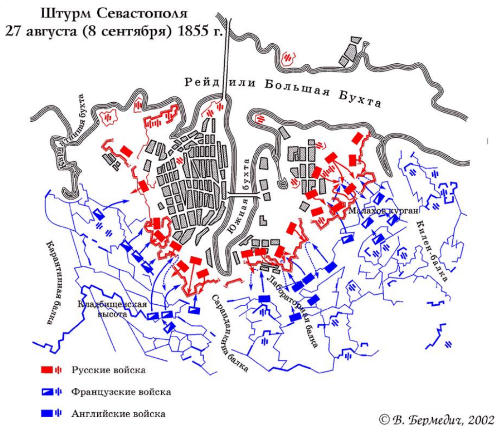
Схема 5.2. Штурм Севастополя 25 августа 1855 г.
